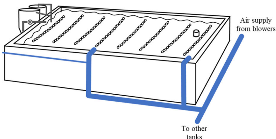
Fig. 1: Sistema de producción con tecnología de biofloc en tanques de madera revestidos de polietileno de alta densidad (6.10 metros x 3.05 metros de dimensiones interiores). El aire de los sopladores suministra dos rejillas de aireación ubicadas en la parte inferior de cada tanque. La bomba de elevación de aire de la corriente lateral mueve el agua del tanque a la primera cámara de sedimentación, que luego fluye por gravedad a la segunda cámara de sedimentación y luego regresa al tanque.
