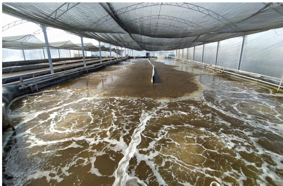
Fig. 2: Vista de un invernadero donde se cría L. vannamei en un sistema BFT en la Estación Marina de Acuicultura (EMA), de donde se obtuvieron los animales y el inóculo de biofloc para este estudio.
