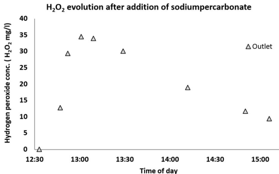
Fig. 2. Concentración de peróxido de hidrógeno medida en relación con la adición de percarbonato de sodio en un estanque de tierra a las 12:35. El volumen del estanque fue de aprox. 100 m 3 ; se añadieron 12 kg de CPS correspondientes a una concentración nominal de H 2 O 2 de 39 mg de H 2 O 2 /L. La temperatura del agua fue de 5-5,5 grados-C y el caudal de entrada fue de aproximadamente 15 L/s.
