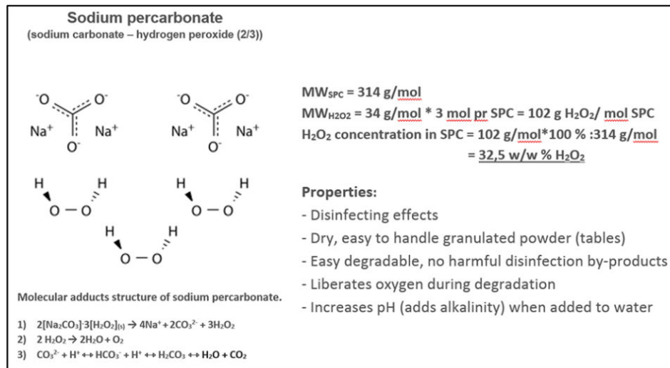
Fig. 1: Estructura molecular y propiedades del percarbonato sódico.
